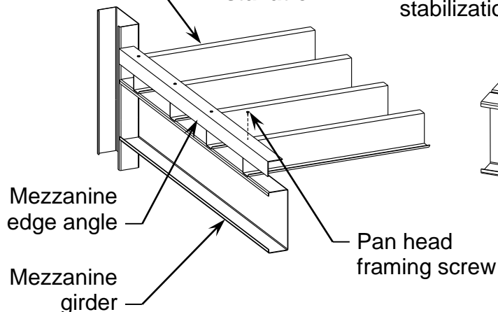
Mezz. Edge Angle Installation
