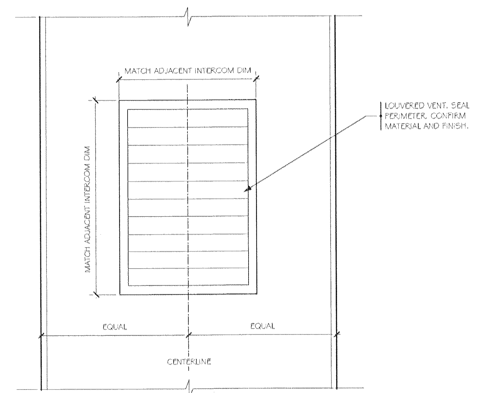
5 ELEVATION DETAIL - VENT SCALE: 3" = 1'-0"
